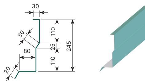
DIỀM CHỐNG TẠT CHÂN NÓC GIÓ FLASHING FOR ROOF MONITOR
