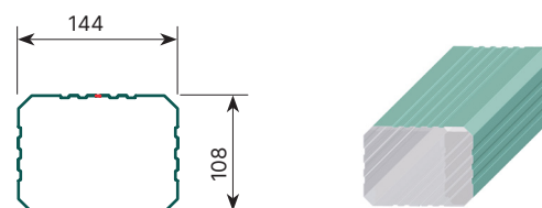
ỐNG XỐI TÔN | DOWNSPOUT
