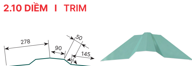
DIỀM ỐP NÓC | RIDGE CAP
