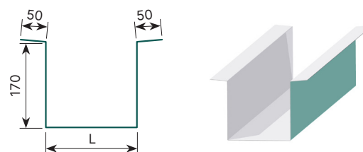
MÁNG XỐI GIỮA | VALLEY GUTTER
