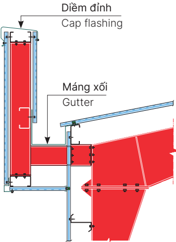
MẶT DỰNG NHÔ RA VERTICAL FASCIA
