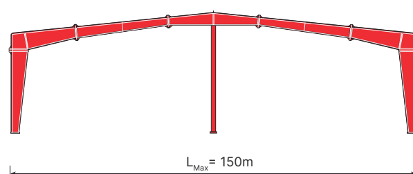
KHUNG KÈO 1 CỘT GIỮA MULTI SPAN 1
