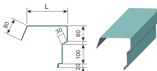
DIỀM MÁI ĐẦU HỒI | GABLE TRIM
