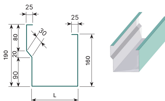
MÁNG XỐI BIÊN | EAVE GUTTER
