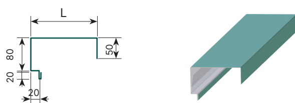
DIỀM ĐỈNH | CAP FLASHING
