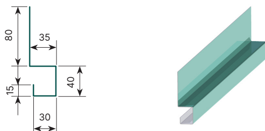
DIỀM CHÂN TÔN | DRIP TRIM
