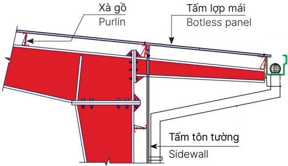
MÁI VƯỢN TƯỜNG BIÊN SIDEWALL ROOF EXTENTION
